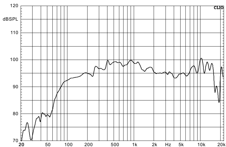
頻響曲綫
